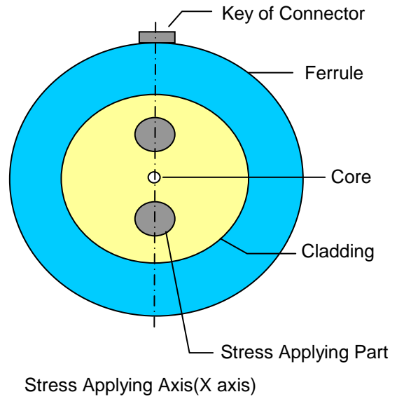
PM- SUS Ferrule
